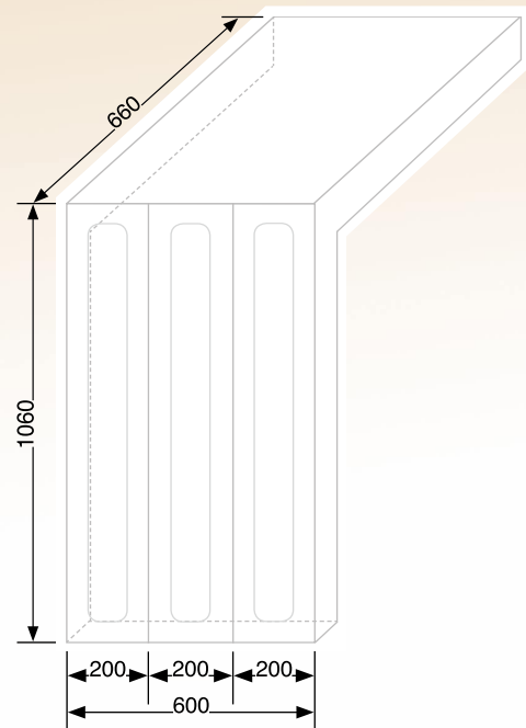
Abb.: Verlängerungspaneel 1:20
