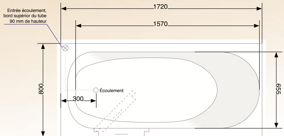
Fig.: Lanzarote Porte à gauche 1:20
