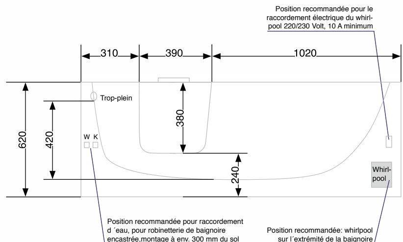
Vue latérale
