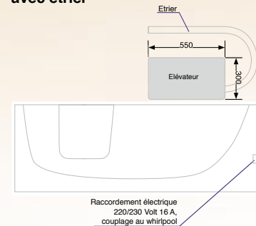
Vue latérale
