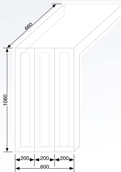
Fig: Panel de prolongación 1:20
