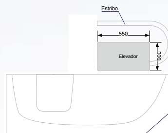
Fig.: Sistema elevador (opcional) con estribo
