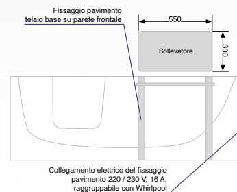
Fig.: Sollevatore (optional) con fissaggio al pavimento
