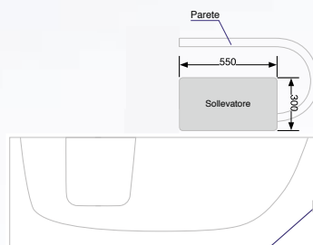
Fig.: Sollevatore (optional) a parete
