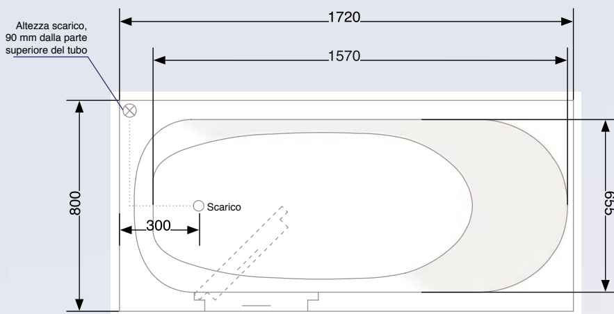
Fig.: Lanzarote Porta sinistra 1:20
