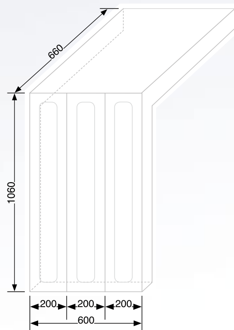
Fig.: Pannello di prolungamento 1:20
