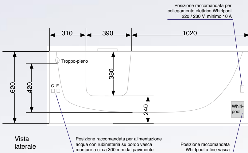
Fig.: Lanzarote Porta sinistra 1:20
